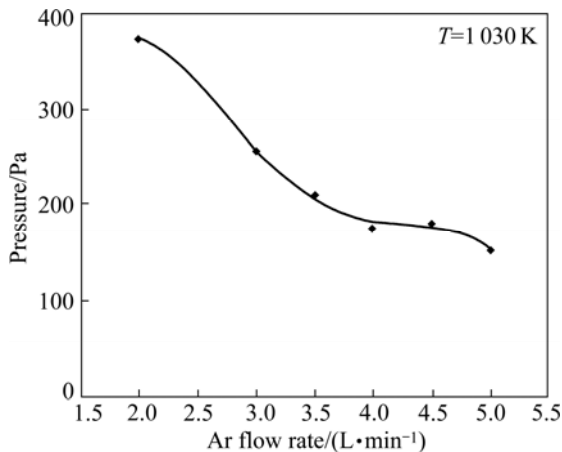
图7 C渣中 ZnCl 2 蒸气压与 Ar 流速的关系
