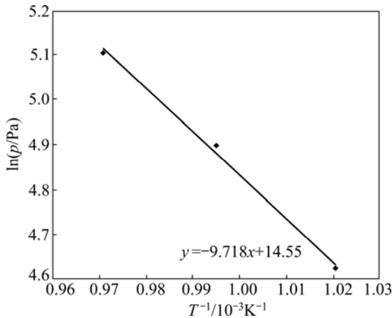
图8 C渣中 ZnCl 2 饱和蒸气压与温度的关系
