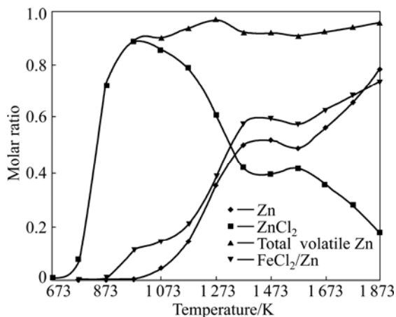
图 6 F 渣中 Zn 挥发物与温度的关系
